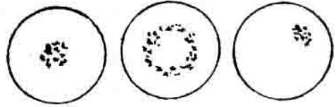
(a) 集中于轴心部位 (b) 分布在1/2R处 (c) 无一定分布规律
