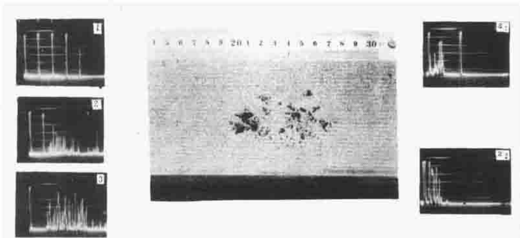
图 1-8 箱体蜂窝缺陷探伤波形
