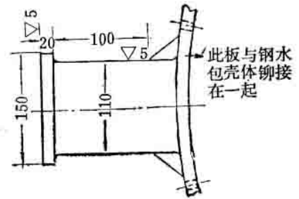
图 1-4 钢水包耳轴尺寸示意图
